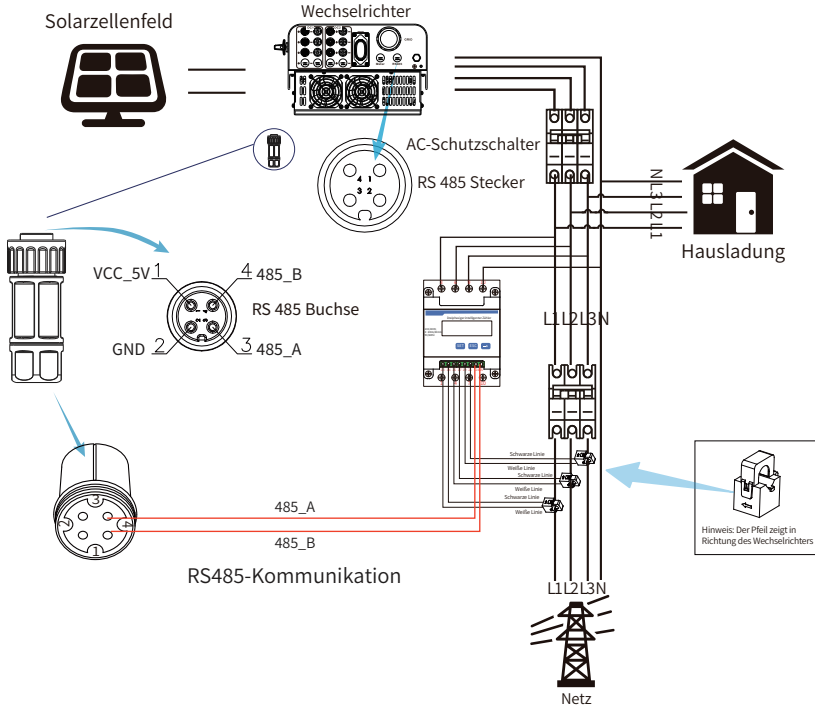
Abb. 7.14 Anschlussplan des CHNT-Zählers
