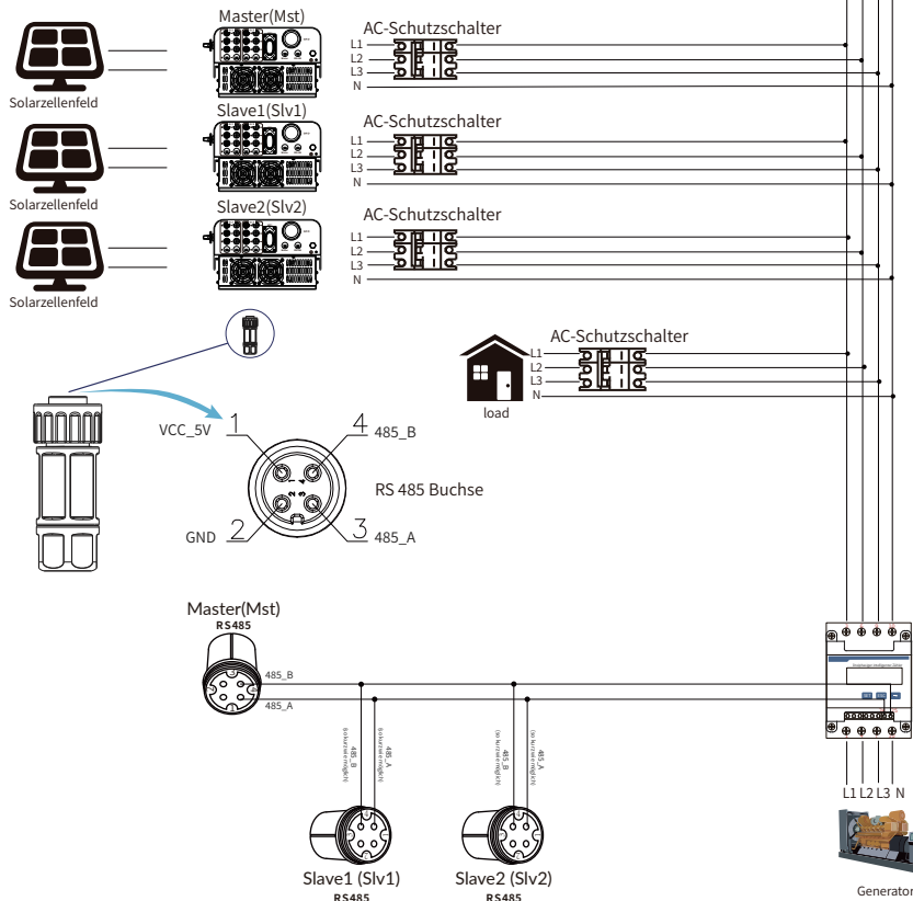
Abb. 7.29 CHNT Anschlussplan (Die Durchleitungstabelle)
