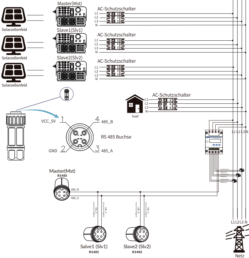
Abb. 7.31 CHNT Anschlussplan (Die Durchleitungstabelle)
