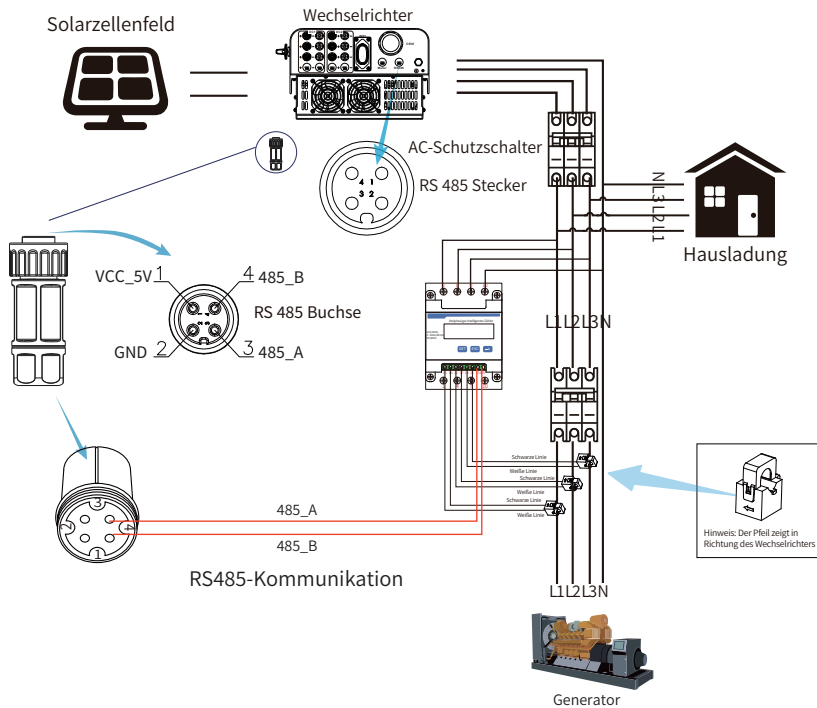
Abb. 7.16 Anschlussplan des CHNT-Zählers
