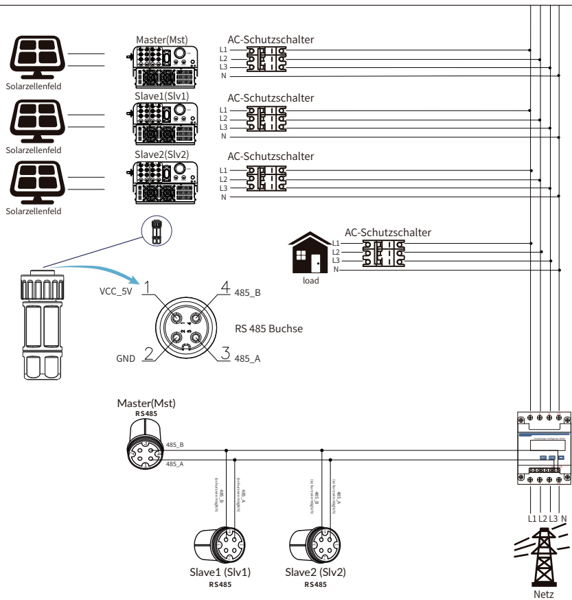
Abb. 7.27 CHNT Anschlussplan (Die Durchleitungstabelle)
