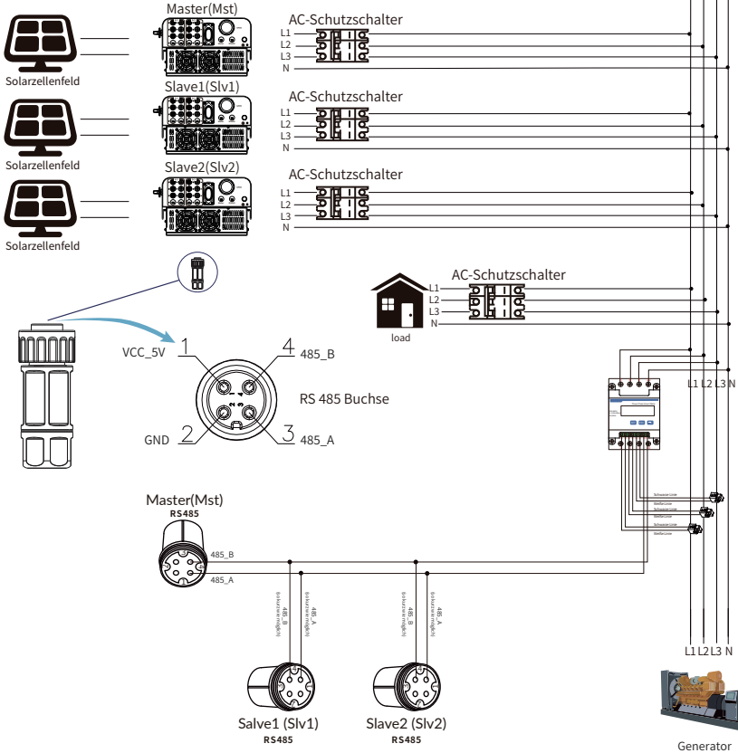
Abb. 7.33 CHNT Anschlussplan (Die Durchleitungstabelle)
