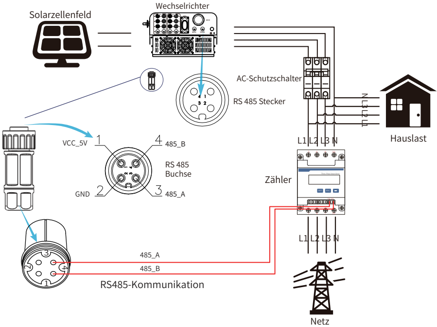
Abb. 7.10 Anschlussplan des CHNT-Zählers
