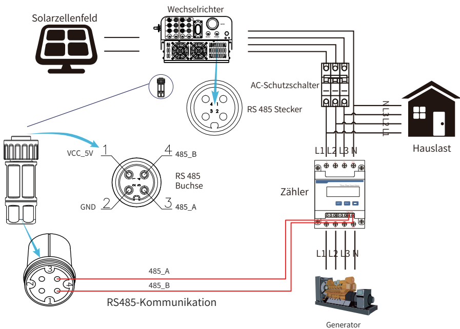
Abb. 7.12 Anschlussplan des CHNT-Zählers
