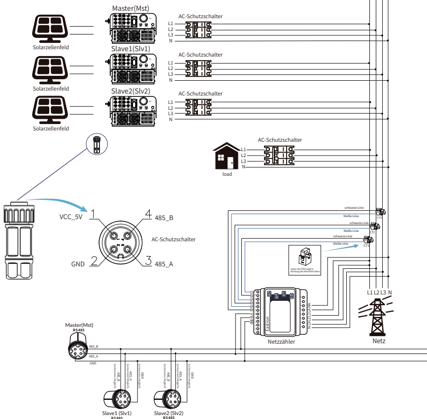
Abb. 7.23 Anschlussplan (Dreiphasenstrom)
