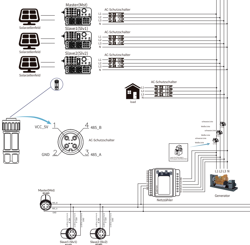
Abb. 7.25 Anschlussplan (Dreiphasenstrom)
